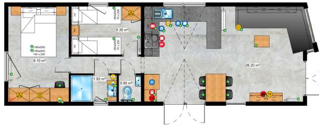
8. 10,86m x 4m / 35ft x 13ft
