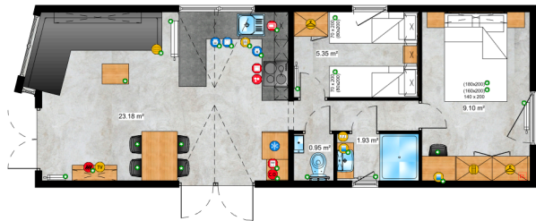
7. 11,66m x 4m / 38ft x 13ft
